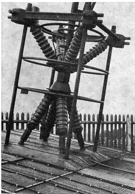
Fig. 6 Bloemberg-Antenne, einer der vier Antennenfüsse
